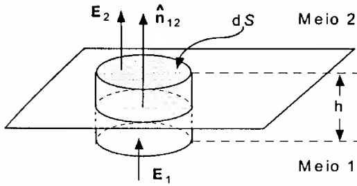
Figura 5.17 Superfície gaussiana
