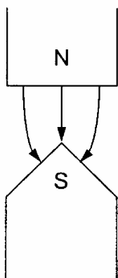
Figura 11.8 Campo B inomogêneo
