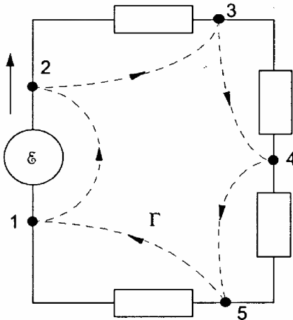
Figura 10.5 Circuito
