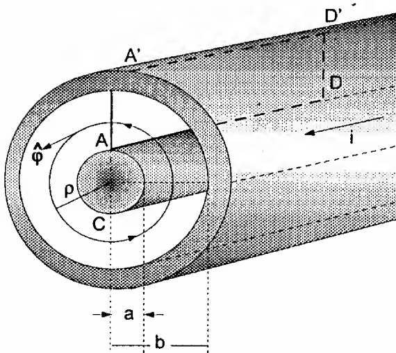
Figura 9.14 Cabo coaxial
