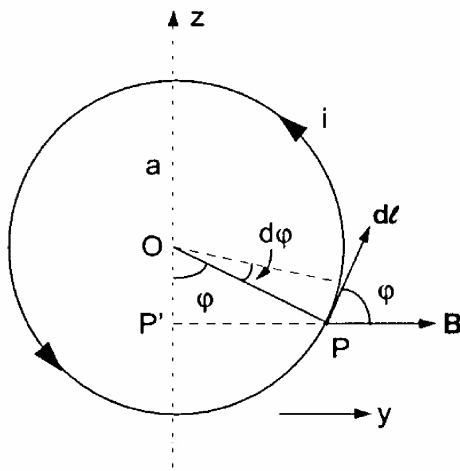
Figura 7.7 Espira circular num campo uniforme
