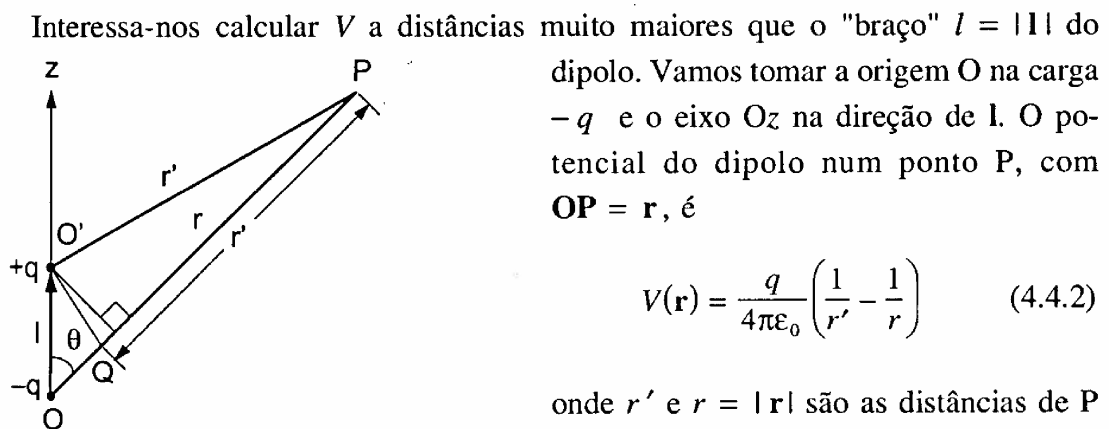
Figura 4.8 Potencial de um dipolo num ponto P distante
