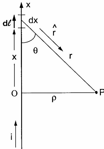
Figura 8.16 Fio retilíneo
