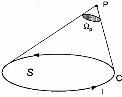
Figura 8.12 Ângulo sólido associado à espira C e ao ponto P
