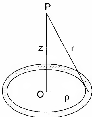
Figura 4.3 Anel carregado
