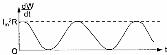
Figura 10.24 Potência instantânea AC dissipada em R
