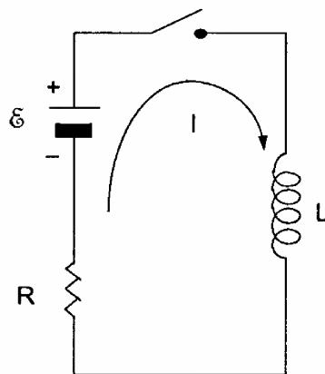
Figura 10.10 Circuito R-L
