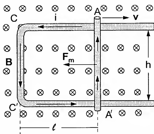
Figura 9.6 Haste metálica móvel sobre trilhos num campo \mathbf{B}
