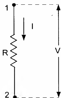
Figura 10.1 Resistor
