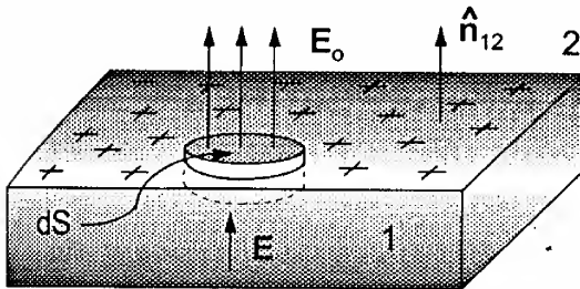
Figura 5.10 Superfície gaussiana
