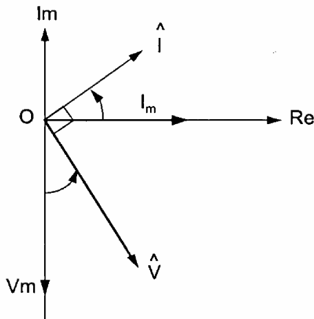
Figura 10.19 Representação c. mplexa de \hat{V} e \hat{I} para um capacitor.
