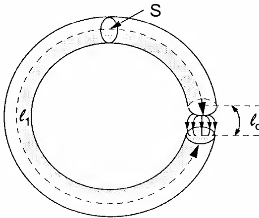
Figura 11.16 Entreferro
