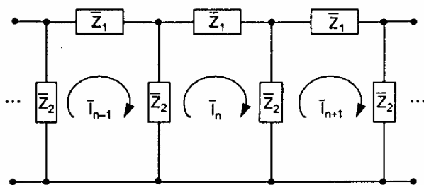
Figura 10.32 Filtro infinito
