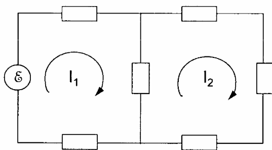
Figura 10.7 Correntes circulantes
