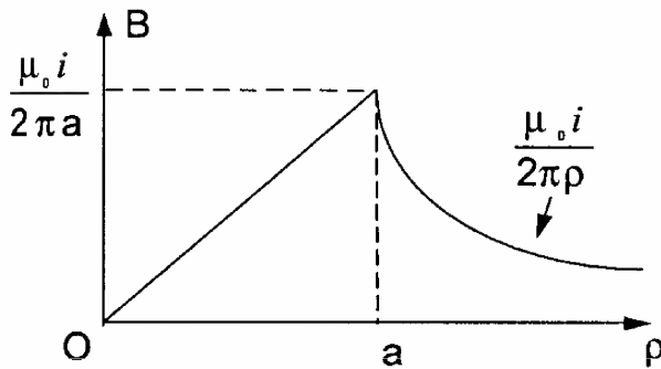
Figura 8.5 Magnitude de \mathbf{B} em função da distância ao eixo
