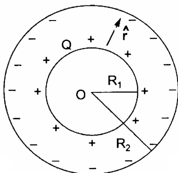
Figura 5.3 Capacitor esférico
