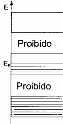
Figura 6.12 Bandas de energia num metal
