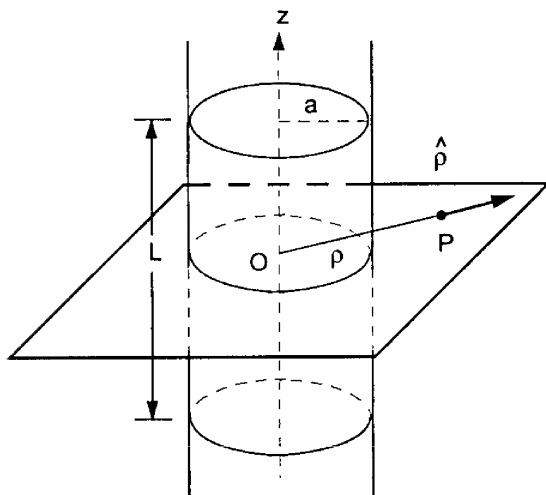
Figura 4.5 Cilindro circular condutor de raio a
