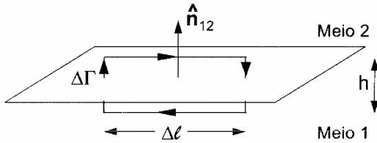
Figura 5.18 Circuito \Delta \Gamma
