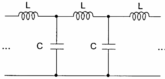
Figura 10.34 Filtro transmissor de baixas frequências
