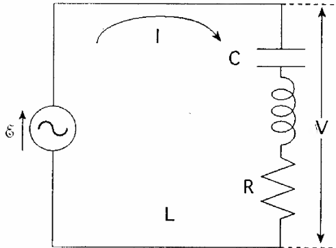
Figura 10.25 Circuito R-L-C com gerador AC
