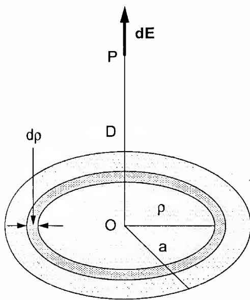
Figura 3.4 Campo de um disco circular
