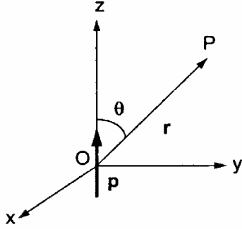
Figura 8.8 Dipolo pontiforme na origem
