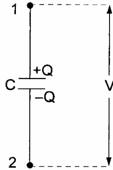
Figura 10.2 Capacitor
