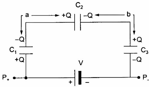
Figura 5.5 Conexão em série
